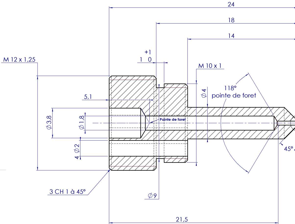
COUPE A-A ECHELLE 6 : 1
