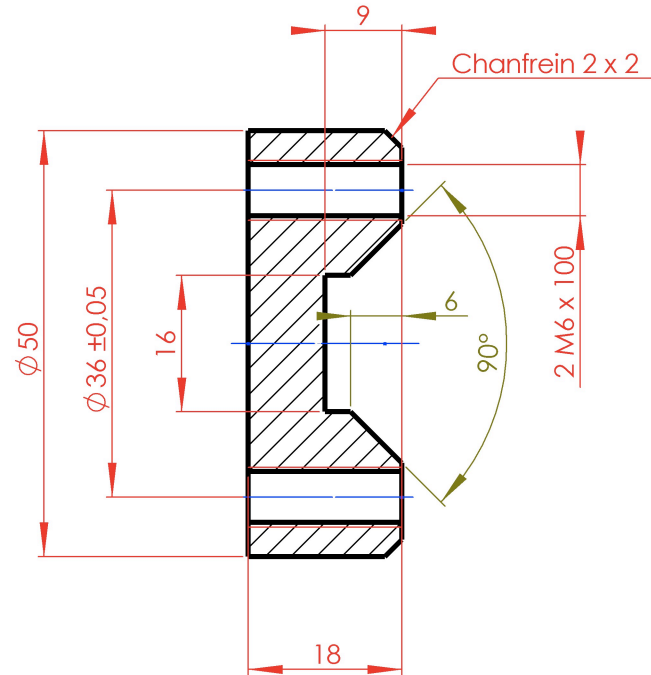
A-A (3 : 2)
