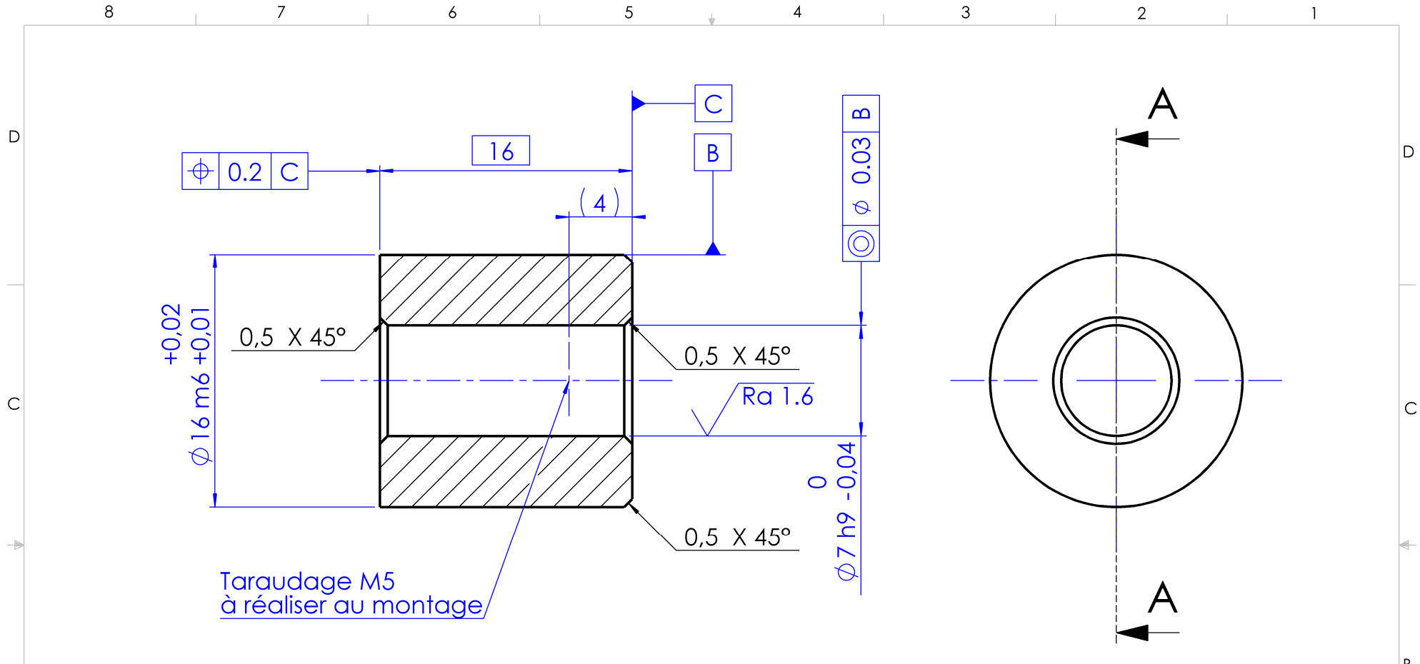
COUPE A-A ECHELLE 3 : 1
