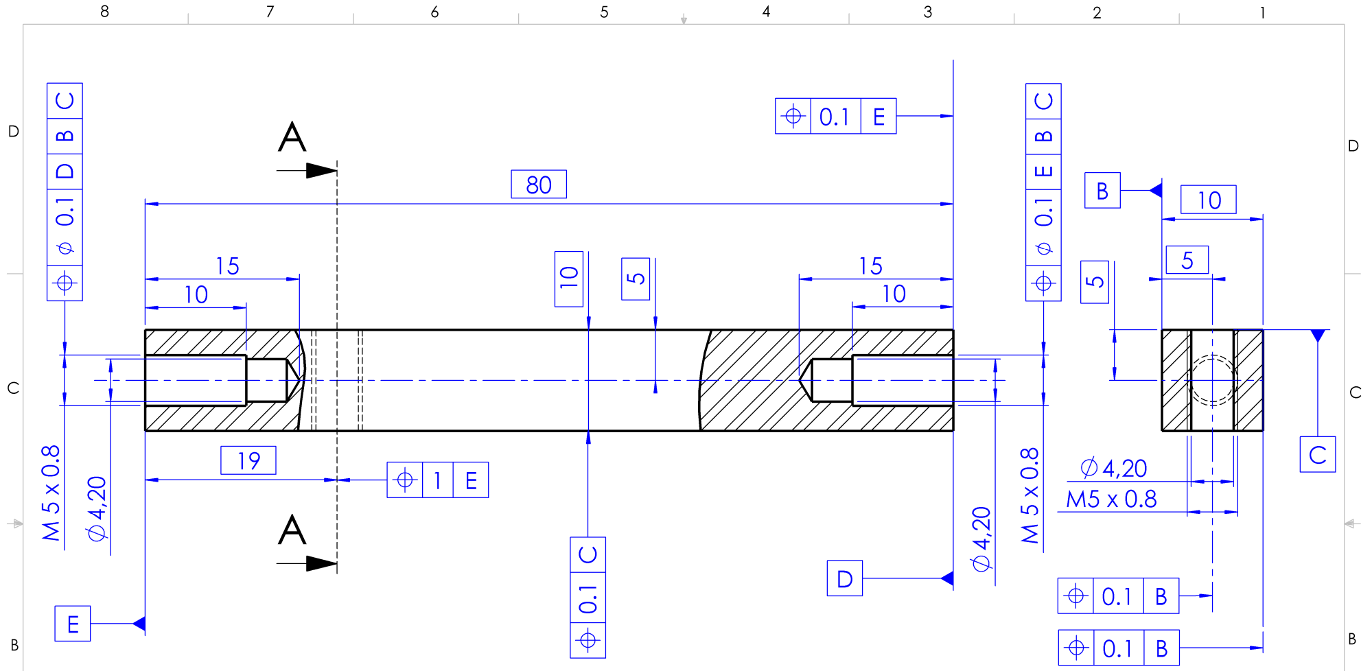
COUPE A-A
