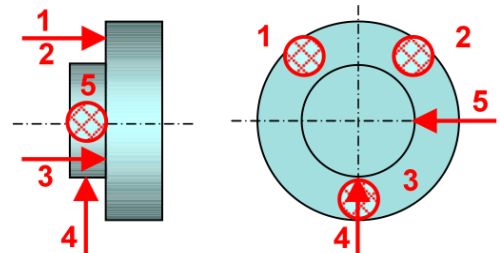
(Tournage) Centrage court en deux vues
