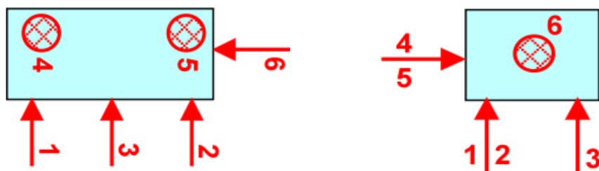
(Fraisage) Isostatisme d'un prisme dans un étau, en 2 vues
